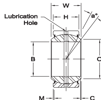
GE..ES-2RS SEALED
