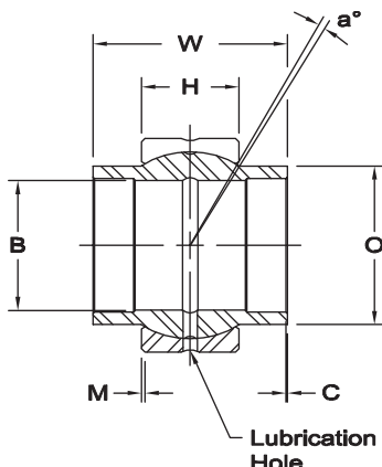
GEWZ..ES OPEN
