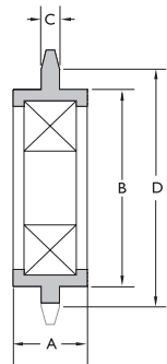
Sprocket
